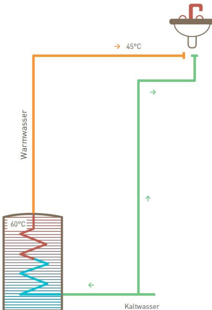
Kombi- / Hygienespeicher
