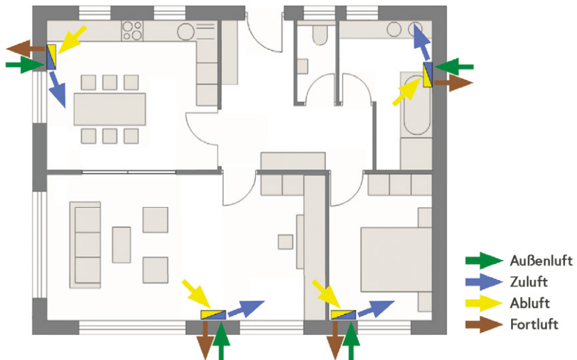
Abb. 2: Lüftungskonzept mit Einzelraumlüftern. Quelle: komfortlüftung.at
